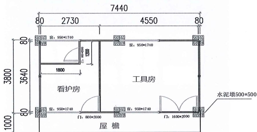
2K*4K*3P(平面图)
